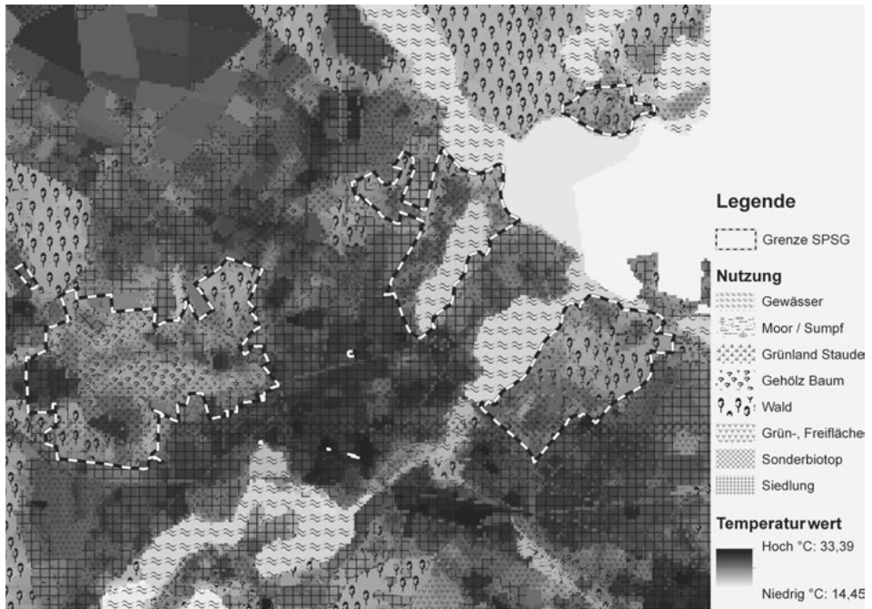
5 Temperaturverteilung errechnet aus Landsat-Daten (2010) in Überlagerung mit Landnutzungsinformation und Flächen der Stiftung Preußische Schlösser und Gärten Berlin-Brandenburg (SPSG).
