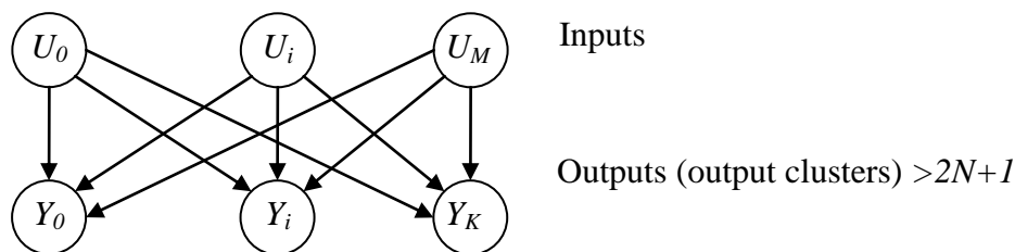
Fig. 2. SOM architecture.
