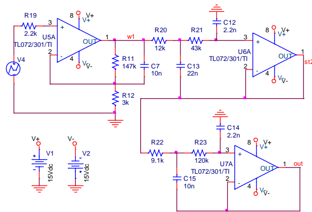
Fig. 12. ECG amplifier.
